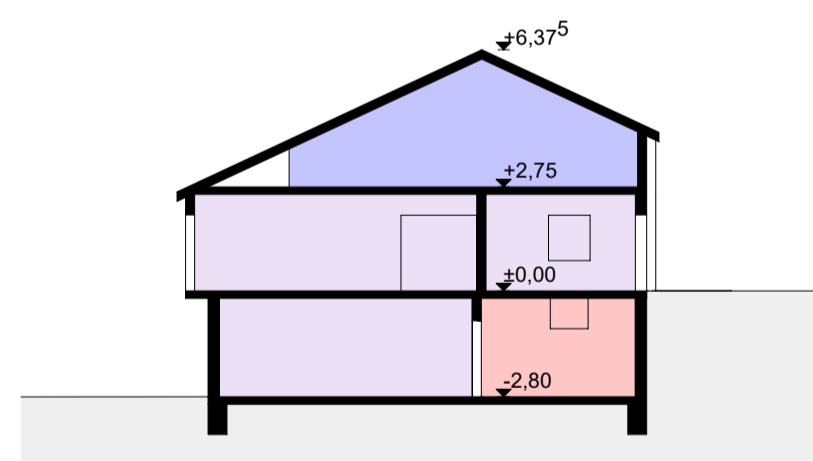
Querschnitt
